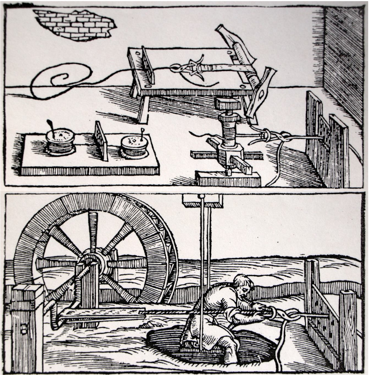
Werkzeuge zum Drahtziehen mit halbautomatisch schließenden Zangen durch Ringmechanik (oben) Drahtziehmühle mit Pleuelstange, Schocke und halbautomatisch schließender Zange durch Ringmechanik (unten)
